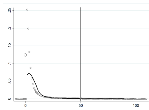
(d) McCrory Test (After Logib)
